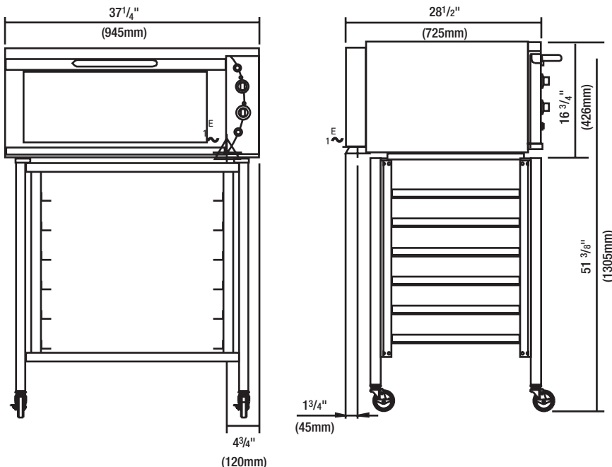
E27MS shown on optional A28CW stand
